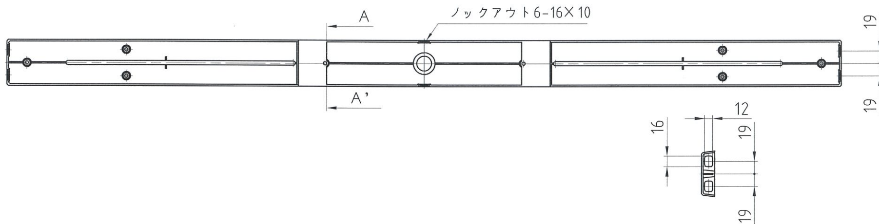
A-A' 断面図
