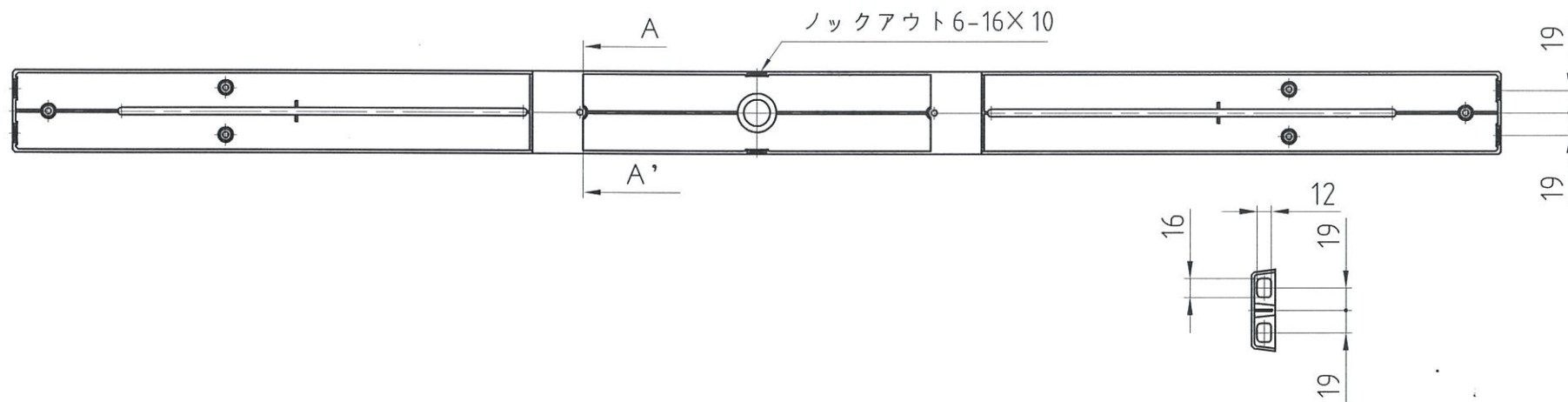
A-A' 断面図
