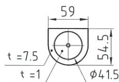
ゴムパッキン詳細 (F)
