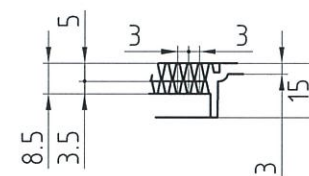
Z部詳細
