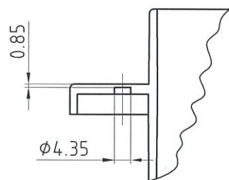
Y - Y 断面図
