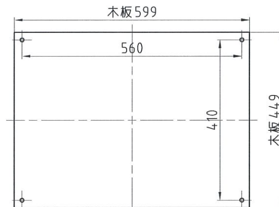
木板ベース
