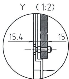
木板ベース
