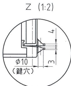
鍵穴詳細
