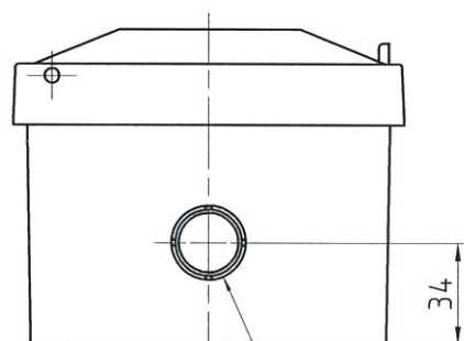
Z矢視図
