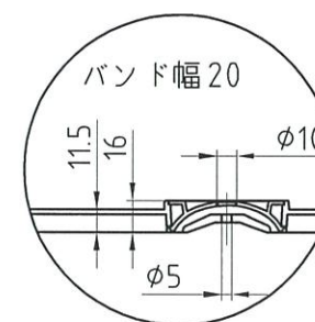
ポール締付部断面
