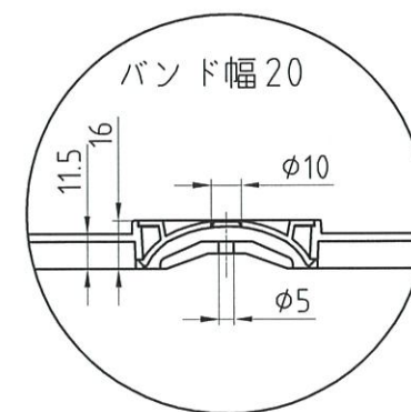
ポール締付部断面
