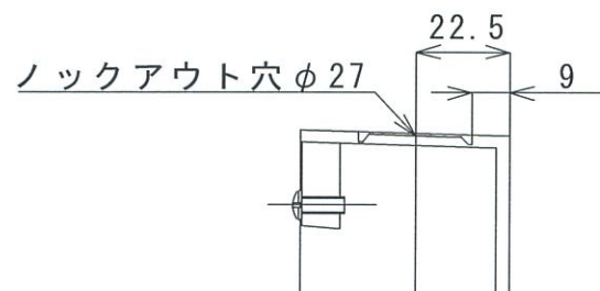
ハブ無し及び1方出ロックアウト部詳細
