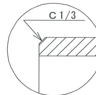
A 部 詳細
